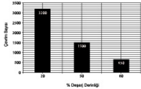
Çevrim Ömrü ve Deşarj Derinliği 25°C
